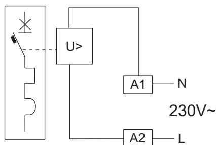
接线图 Wiring diagram
